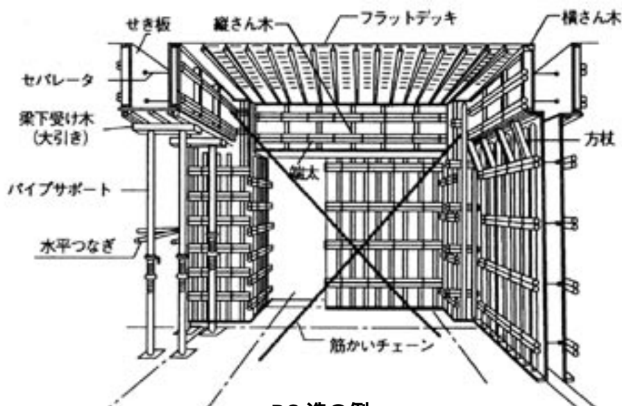
RC 造の例
