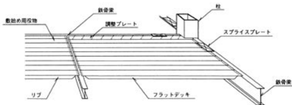
S 造の例
